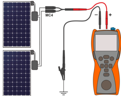
R ISO -Messung in PV-Anlagen mit Optimierern
