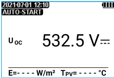
Messergebnis bei inaktiver Verbindung mit IRM-1
